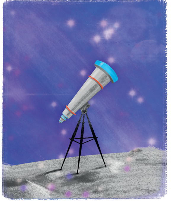
Teleskop
