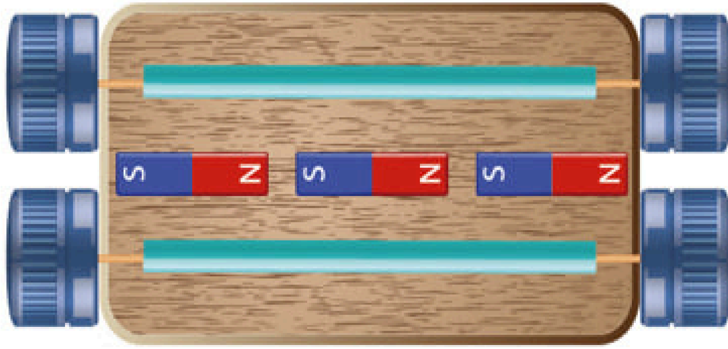
Şekil 1-A Alttan görünüm
